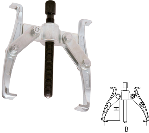
S Tipi Çektirme (İki Kollu) S Type Puller (Two Arms)
