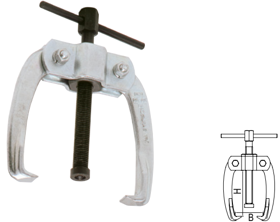
Batarya Çektirme (İki Kollu) Battery Puller (Two Arms)
